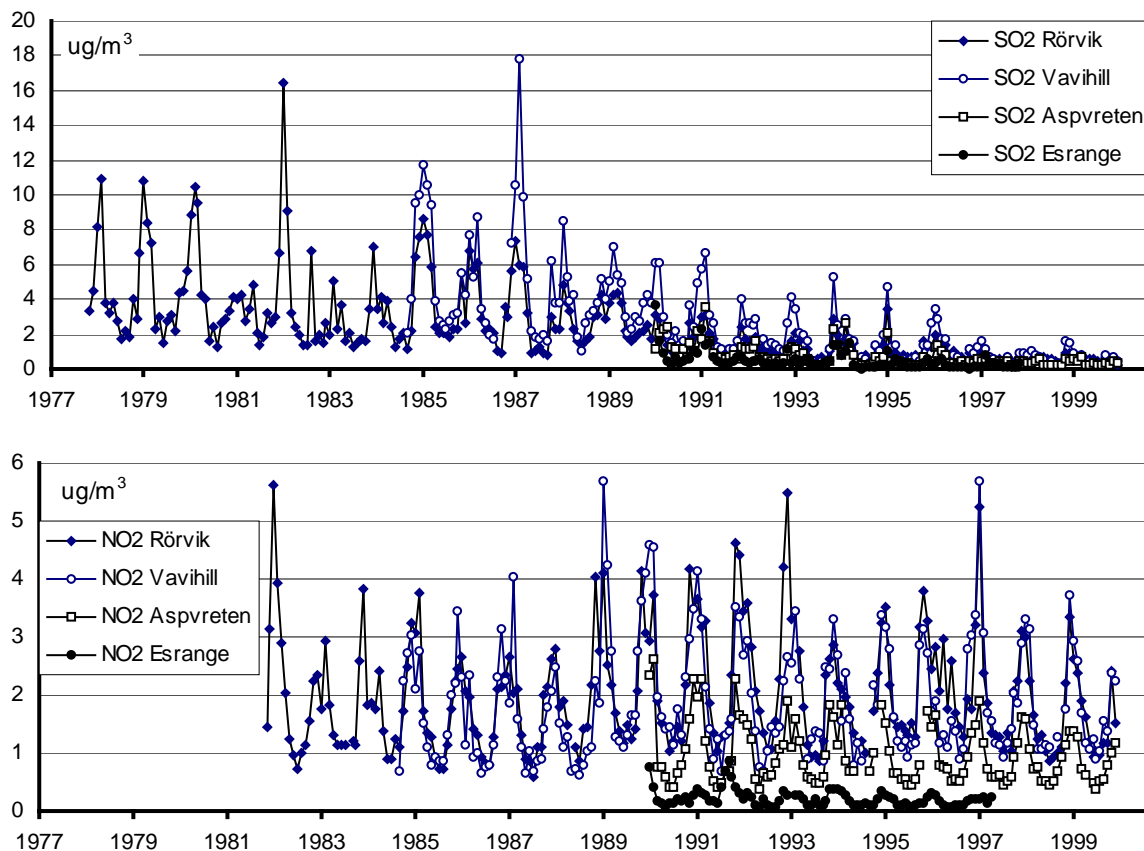
Figur 11. Månadsmedelvärden för luftens innehåll av svaveldioxid, (SO 2 ), kvävedioxid (NO 2 ) och ozon (O 3 ) på fyra EMEP-lokaler i Sverige; Vavihill i centrala Skåne, Rörvik söder om Göteborg, Aspvreten öster om Nyköping samt Esrange öster om Kiruna. Observera att stationernas mätningar startar olika år.
