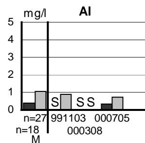
Figur 5. Depositions- och markvattendata från Kallgårdsmåla, K 10.
