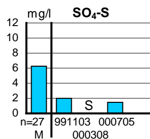
Figur 5. Depositions- och markvattendata från Kallgårdsmåla, K 10.
