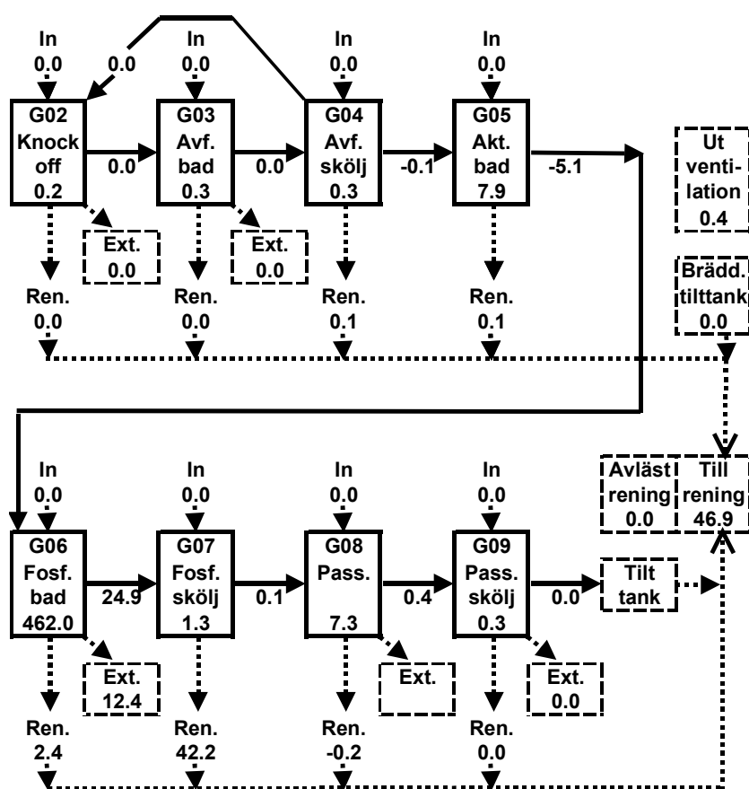
Figur 4.11 Exempel på förenklat flödesschema för nickel, enhet mg/m 2 . Negativa värden avser att flödet går motsatt pilens riktning. Nickelflödet från G07 är troligen överskattat. Ett mer troligt värde på nickelflödet från jonbytareluaten ska därför vara ca 25 mg/m 2 (jämför ingående mängd till G07). Detta påverkar även det summerade flödet till reningsverket som bör justeras ned i motsvarande grad (till ca 30 mg/m 2 ), se även stycket balans i nickelavsnittet.
