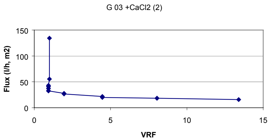
Figur 5.31 b) Försök 3, rest från försök 2, kört igen vid senare tillfälle, uppkoncentrering
