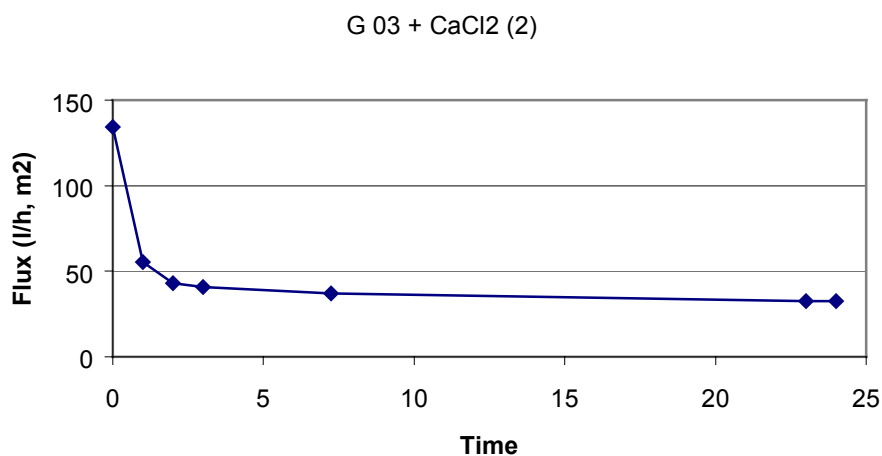
Figur 5.31 a) Försök 3, rest från försök 2, kört igen vid senare tillfälle, VRF 1
