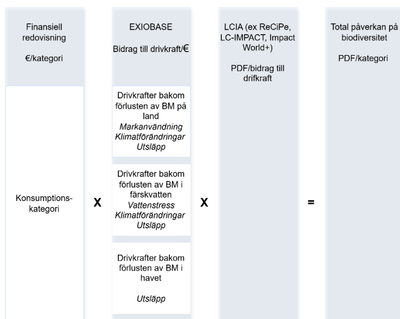
Figur 3. Illustration av hybridmetoden som kombinerar LCA och EEIOA.
